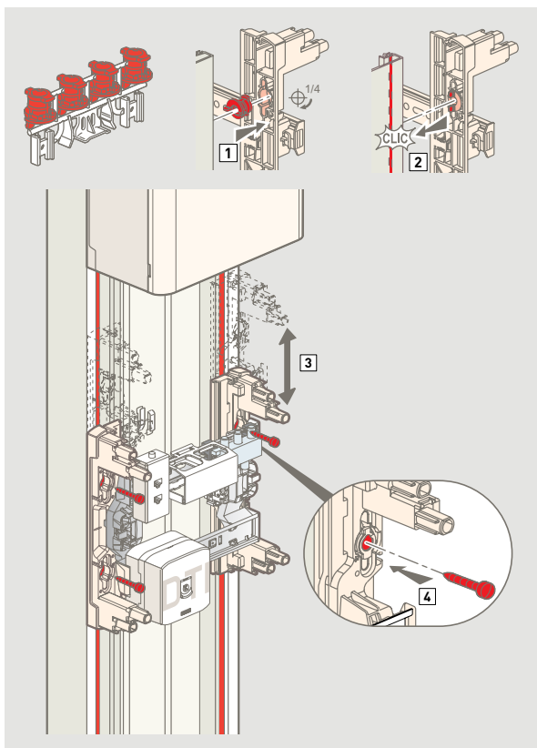
2 - Montez la cloison de séparation.
