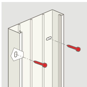
1 - Fixez la goulotte au mur.
