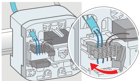
2 - Passez le câble téléphonique et rabattez le levier pour assurer la connexion.
